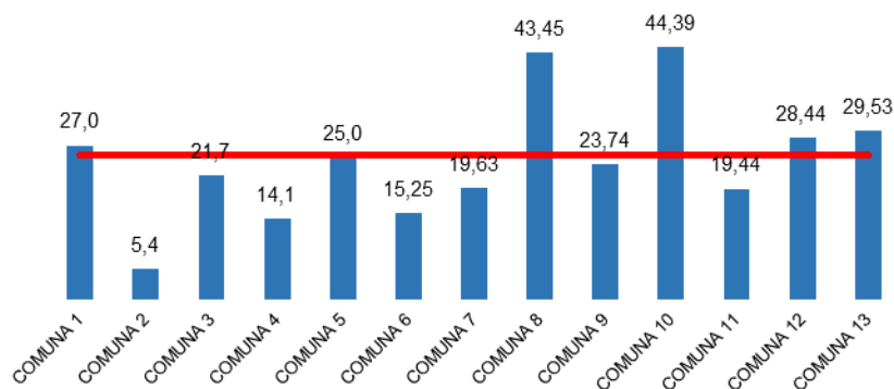
Gráfico 10. Índice Aéxico de vivienda, Ibagué, primer muestreo del año 2017
